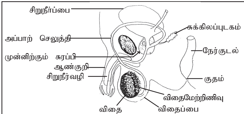
உரு 9.3 ஆணின் இனப்பெருக்கத் தொகுதி
